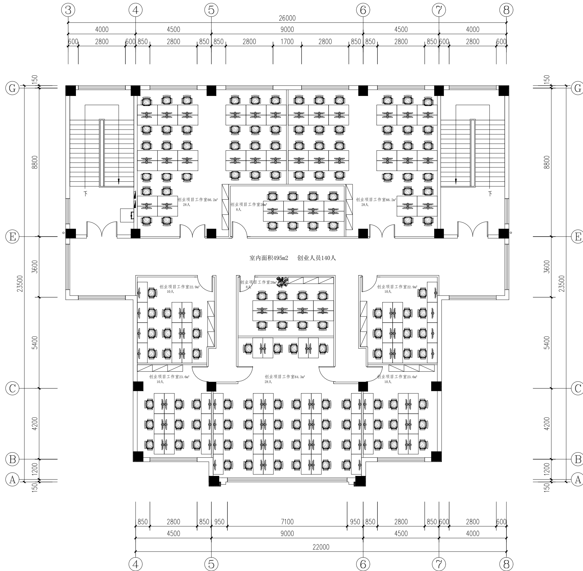
三层平面布置图 1:150
